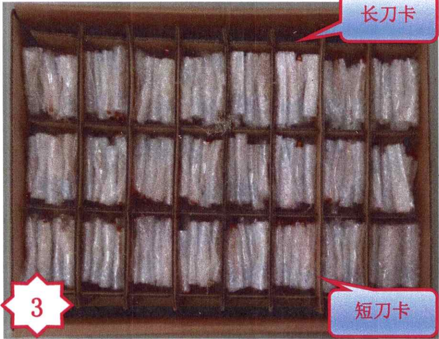
图三, 将 PA2192 按照每层 192 个, 每箱 3 层的方式进行包装, 同时在底层和每层的顶部放一块隔板, 共 4 块隔板。
